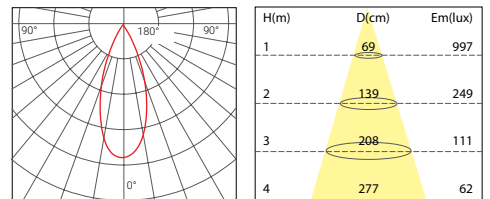
7W 40° 3000K
