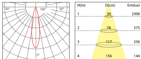
7W 24° 3000K
