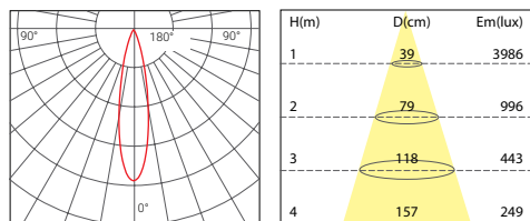
11W 24° 3000K
